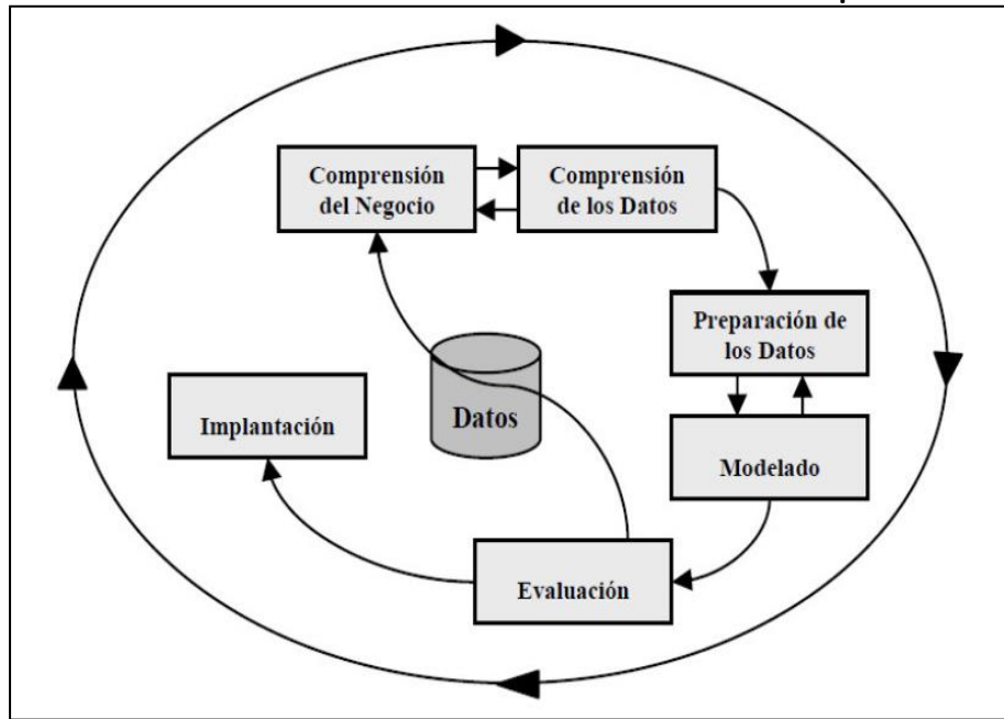
Ilustración 1. Metodología CRISP-DM
